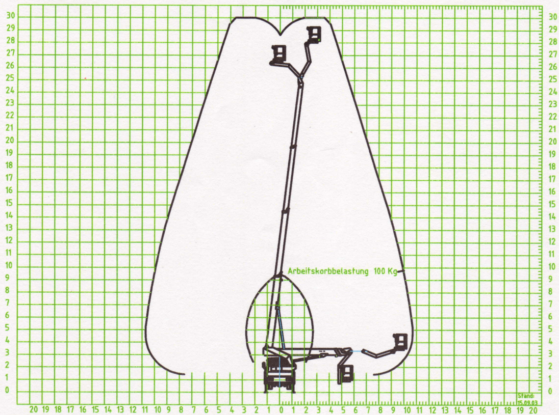
Kennfeld TKA 30 KS Abstützung schmal/schmal
