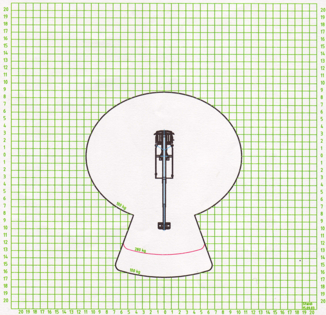
Kennfeld TKA 30 KS Abstützung schmal/schmal
